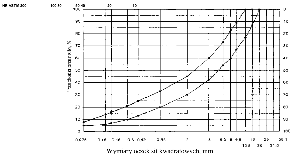
Rys. 13. Krzywe graniczne uziarnienia mieszanki mineralnej BA od 0 do 16 mm do warstwy wyrównawczej nawierzchni drogi o obciążeniu ruchem od KR3 do KR6
