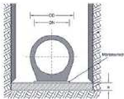
zdjęcie 1 podbudowa typ III
