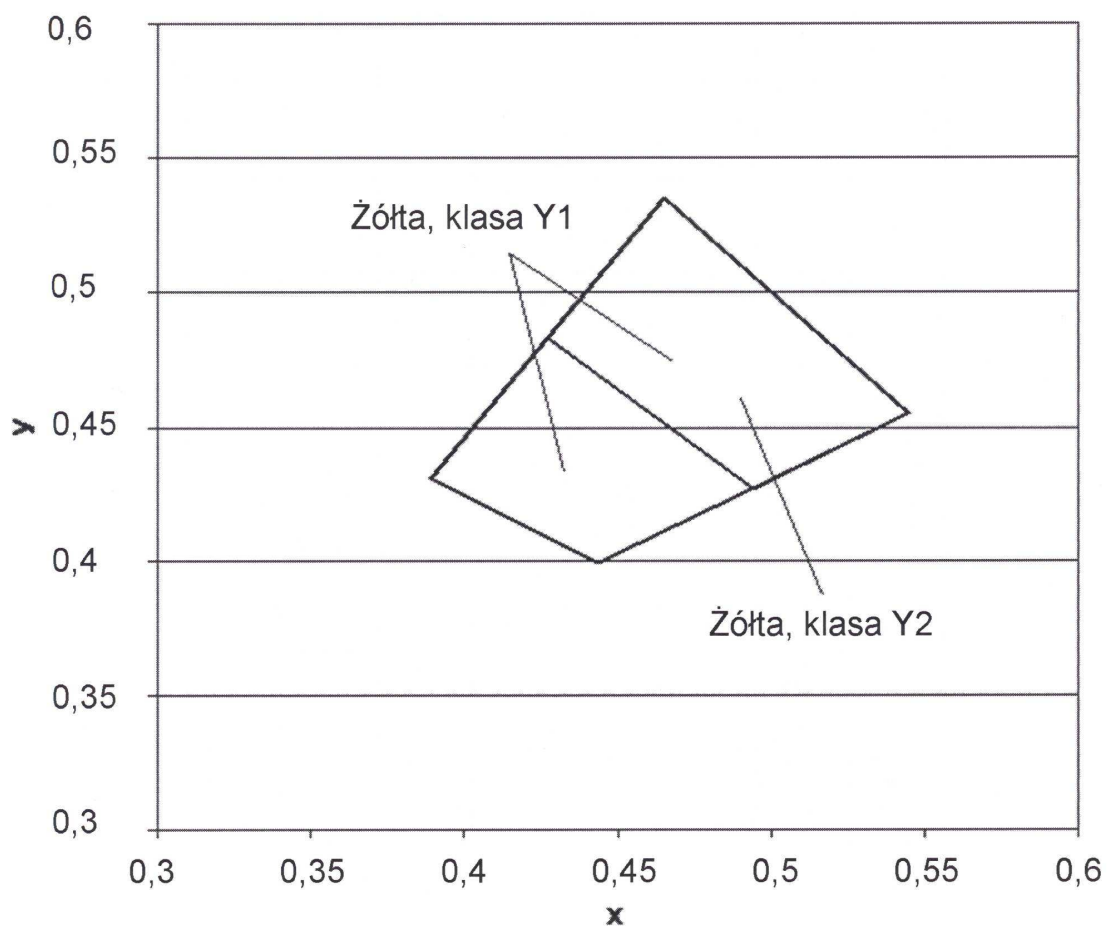
Rys.2. Współrzędne chromatycyjnosc x, y dla barwy żółtej oznakowania
