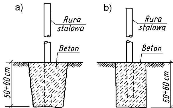
Rys. 4. Przykład ustawiania słupków ogrodzenia (wg [6])
