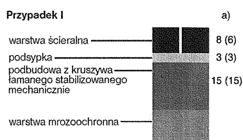
2.2. Konstrukcja nawierzchni dla kategorii ruchu R 1 – grubość warstwy w [cm]
