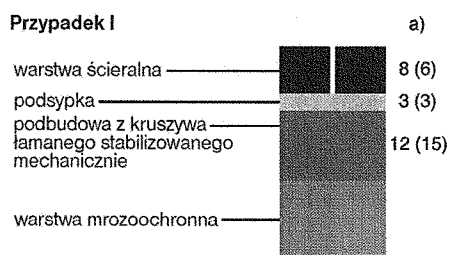
2.1. Konstrukcja nawierzchni dla kategorii ruchu R 0 – grubość warstwy w [cm]
