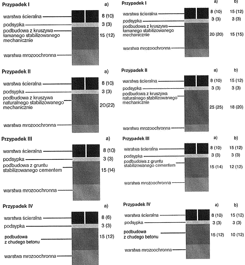
2.3. Konstrukcja nawierzchni dla kategorii ruchu R 2 – grubość warstwy w [cm]
