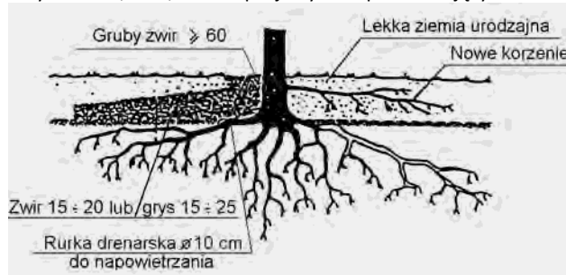
Rys. 4. Pień drzewa obsypany na wysokość 0,2 \div 0,5 m ze specjalnymi napowietrzającymi warstwami żwirowymi
