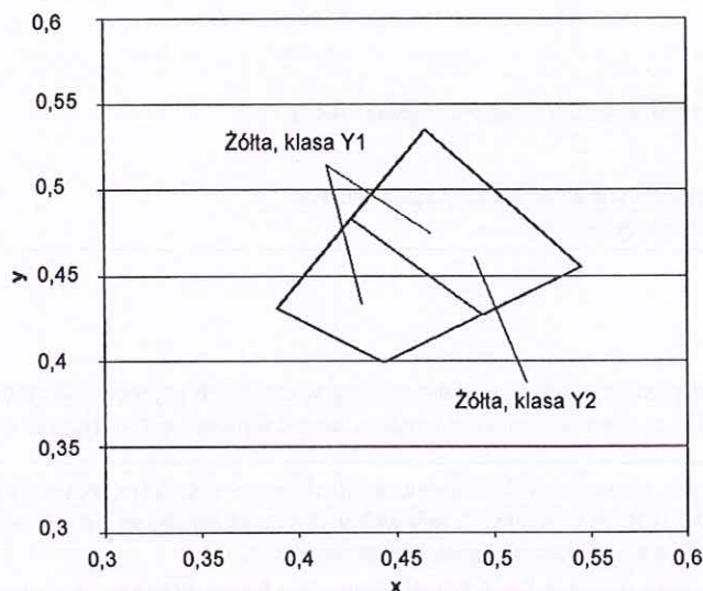
Rys.2. Współrzędne chromatycznosci x,y dla barwy żółtej oznakowania
