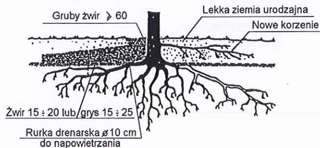
Rys. 4. Pień drzewa obsypany na wysokość 0,2 \pm 0,5 m ze specjalnymi napowietrzającymi warstwami żwirowymi
