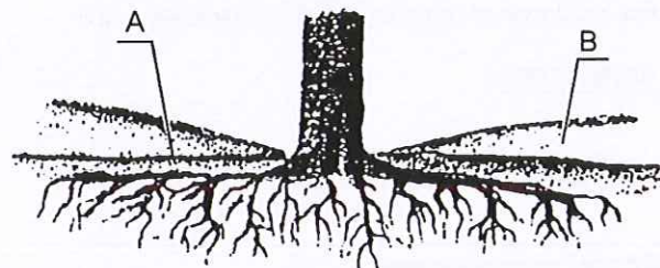
Rys. 3. Niecka o łagodnym pochyleniu, dostosowująca drzewo do otaczającego terenu podwyższonego o 0,2 \pm 0,4 m
