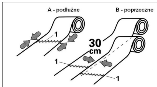
Rys. 3. Łączenie pasm siatki A - łączenie podłużne pasm (pręty płaskie obu siatek blisko siebie) B - łączenie poprzeczne pasm (pręty płaskie obu siatek odsunięte od siebie) 1 - Wzmacniający siatkę poprzeczny pręt płaski
