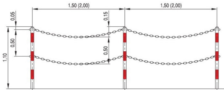
Wzór ogrodzenia łańcuchowego U-12b
