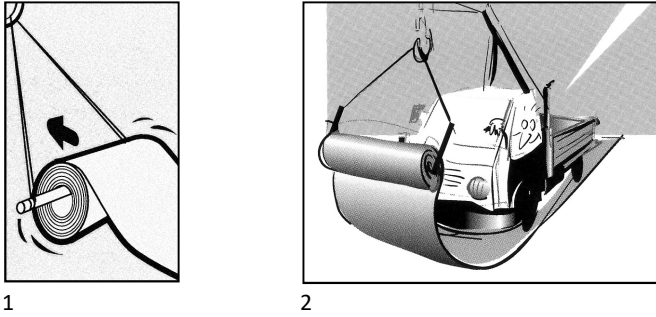
1 2 Rys. 2. Ułożenie siatki na podłożu 1 – Rolka siatki umocowana na wysięgniku pojazdu, 2 – Ciężki pojazd rozwijający siatkę przeciwbieżnie do kierunku jej zwinięcia
